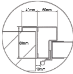
Присоединительные размеры
